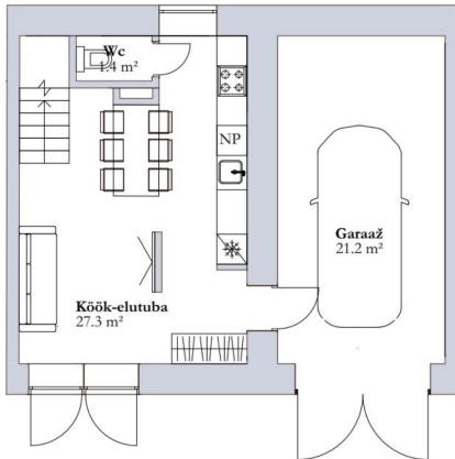
1.korruse illustratiivne plaan
