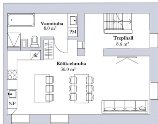
2.korruse illustratiivne plaan
